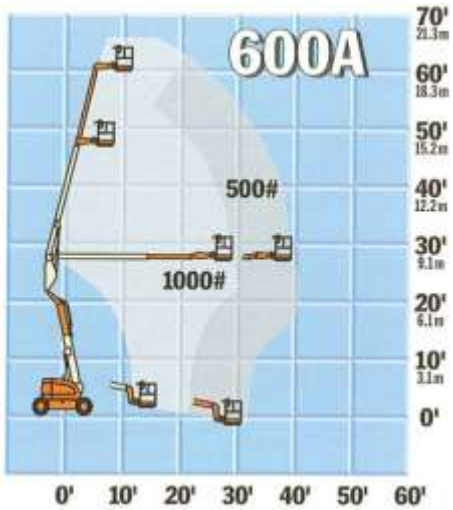
JLG 600A Manlift #1976
